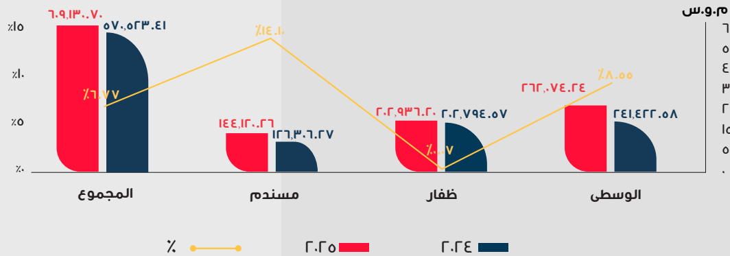
الشكل (١٢): الطاقة الفعلية المنتجة لكل منطقة (بالميجاواط /ساعة)
