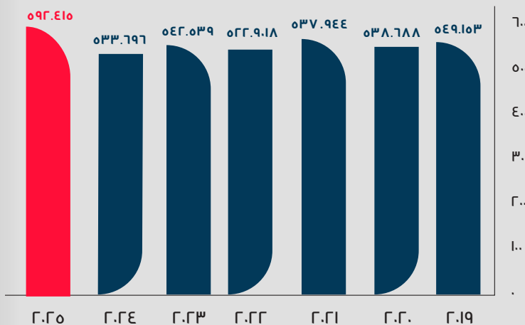
الشكل (٦): إجمالي الكهرباء المُنتجة بمحطة لمزيونة للطاقة الشمسية (ميجاواط/ ساعة)
